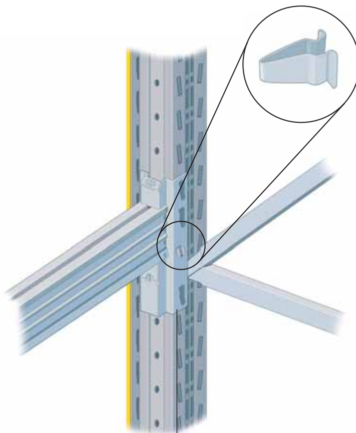
5 Antisgancio trave variant Locking clip Anti-décrochage poutre VARIANT Loslösicherung VARIANT - Träger Antidesenganche vigas variantes
