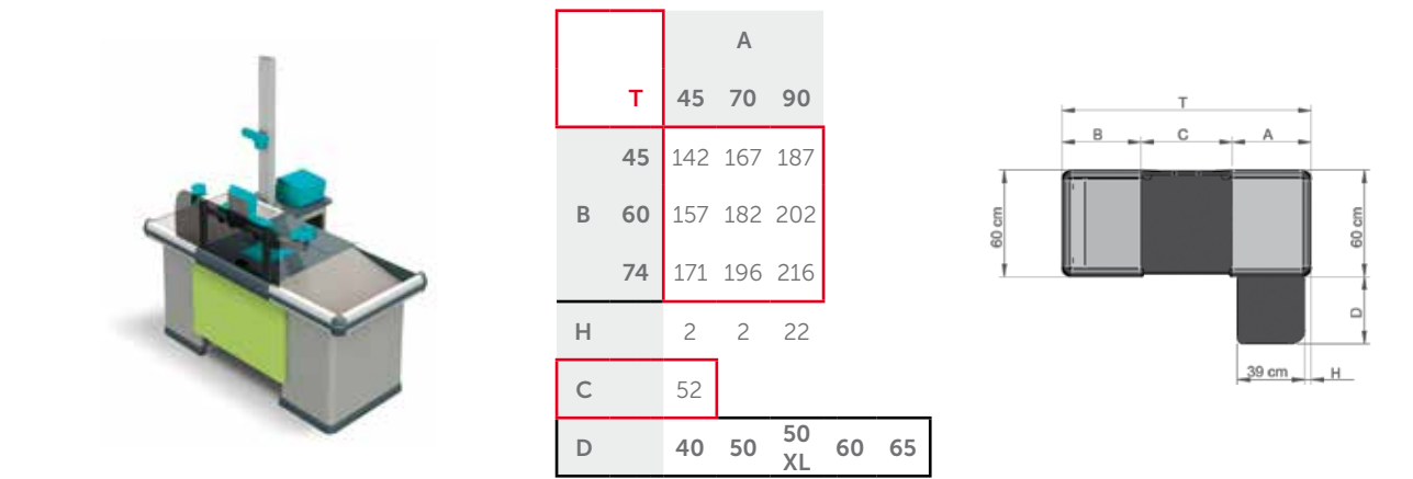
SINGOLO VASCA LARGA - STATICO • NARROW SINGLE BASIN - FRONT CABINET - STATIC
