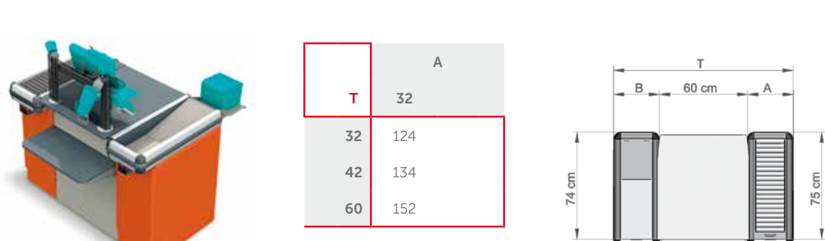
SINGOLO VASCA LARGA - RULLIERA • SINGLE VERSION - ROLLER TABLE
