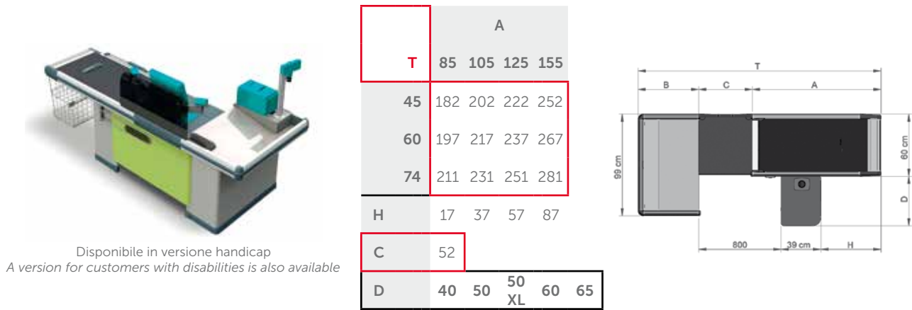
SINGOLO VASCA LARGA - RULLIERA • WIDE BASIN - SINGLE VERSION - ROLLER TABLE
