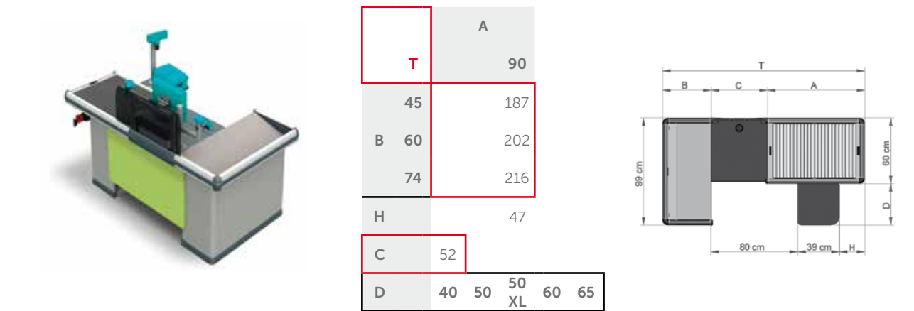
SINGOLO VASCA LARGA - STATICO • WIDE BASIN - SINGLE VERSION - STATIC
