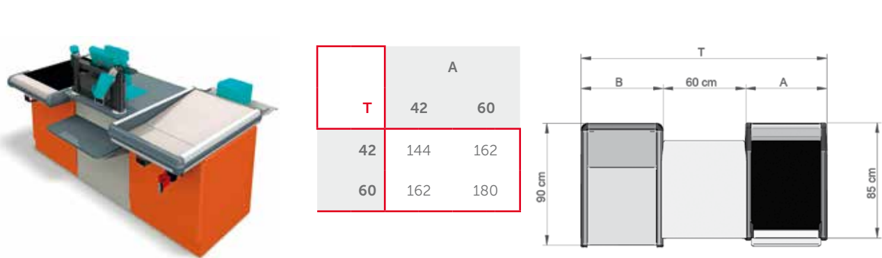
SINGOLO VASCA LARGA - MOTORIZZATO • SINGLE VERSION - POWERED
